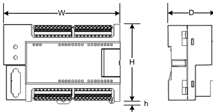
图 1 模块尺寸图
