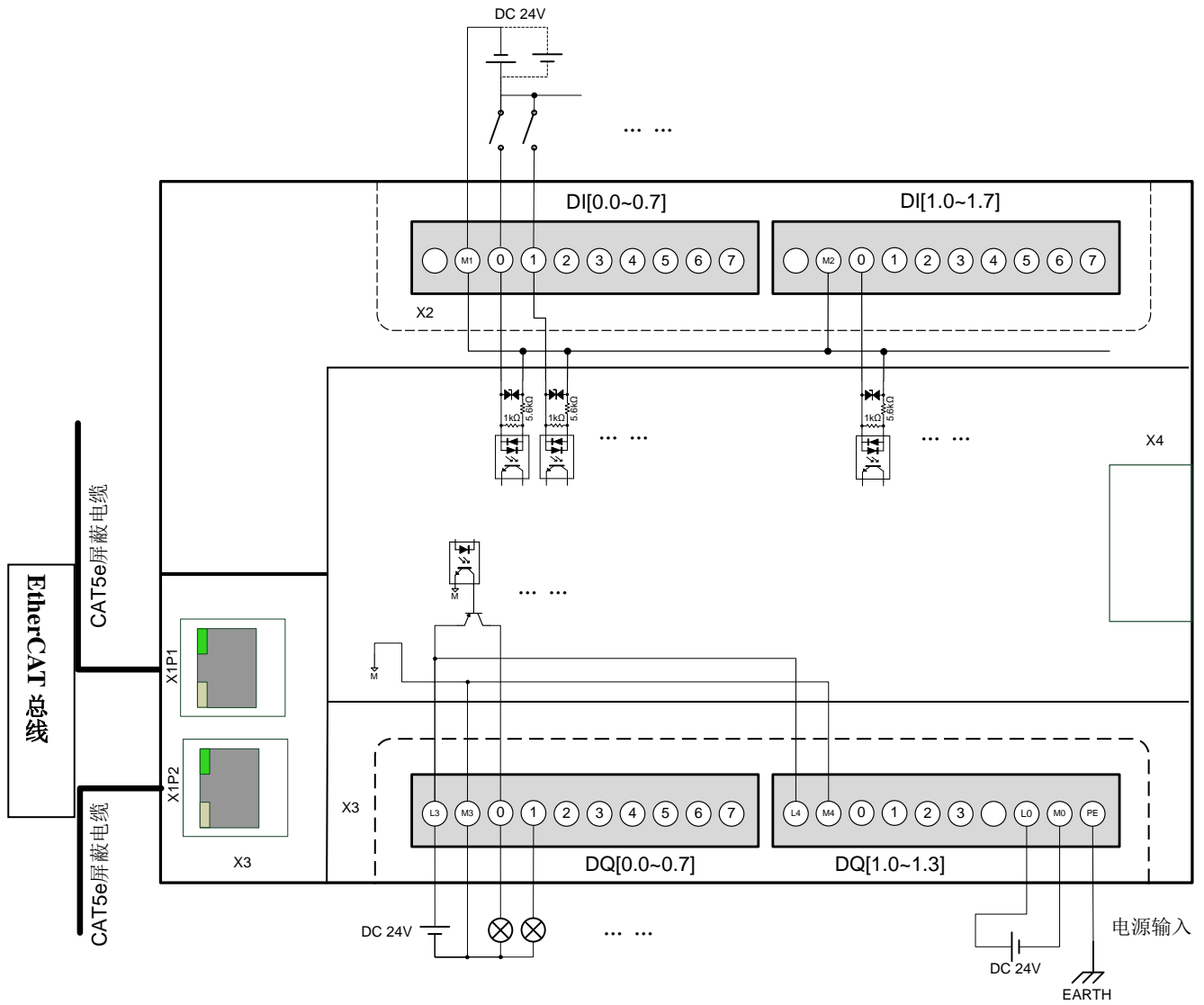
图 3 模块接线图
